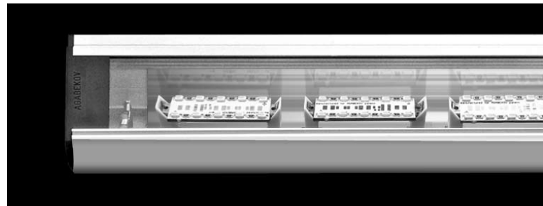
Photo: LL3AL IP65 avec AGA-LED® B-10 lighting units rigid loop connector / 24V / 1W
